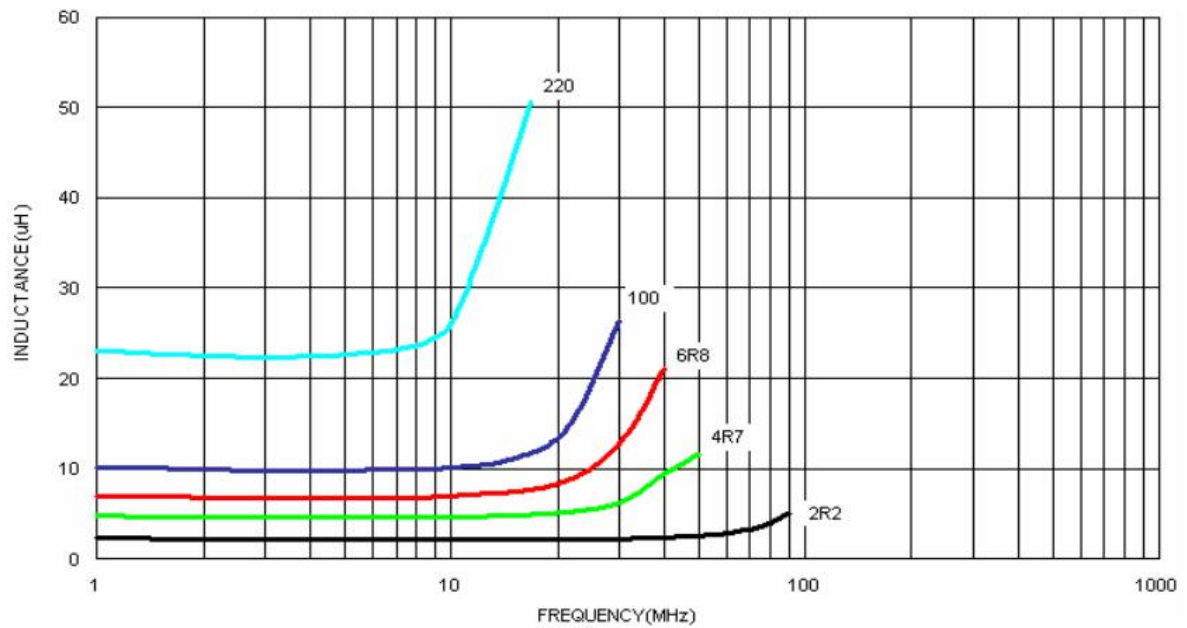
PWFI 2012(0805)
