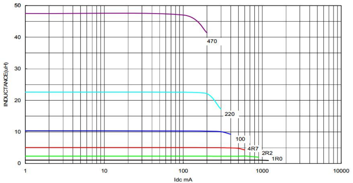
PWFI 2012(0805)
