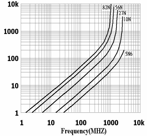
PFCI 2012(0805) TYPE
