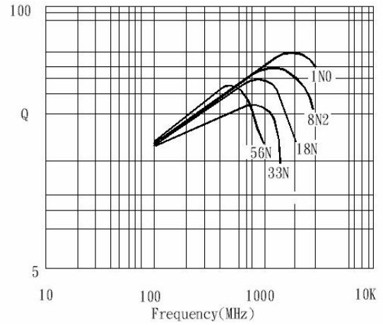
PFCI 2012(0805) TYPE
