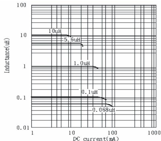
PFFI 1608(0603) TYPE
