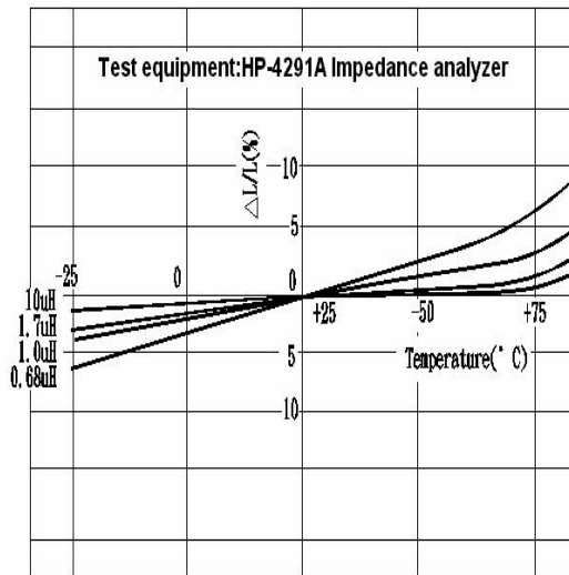
PFFI 1608(0603) TYPE
