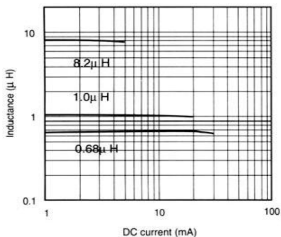
PFFI 1005(0402) TYPE
