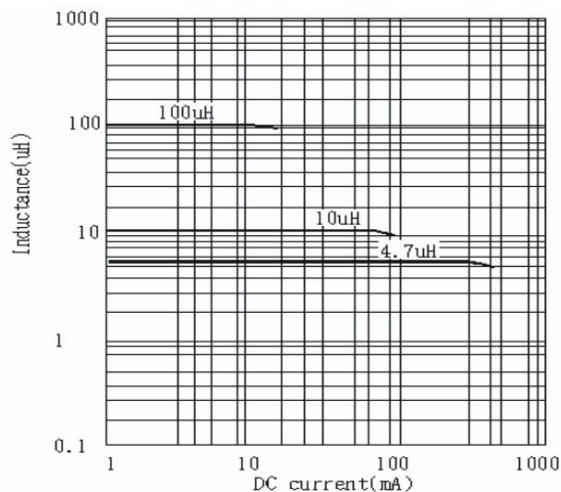
PFFI 4532(1812) TYPE
