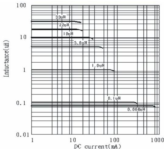
PFFI 2012(0805) TYPE
