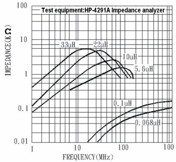
PFFI 2012(0805) TYPE
